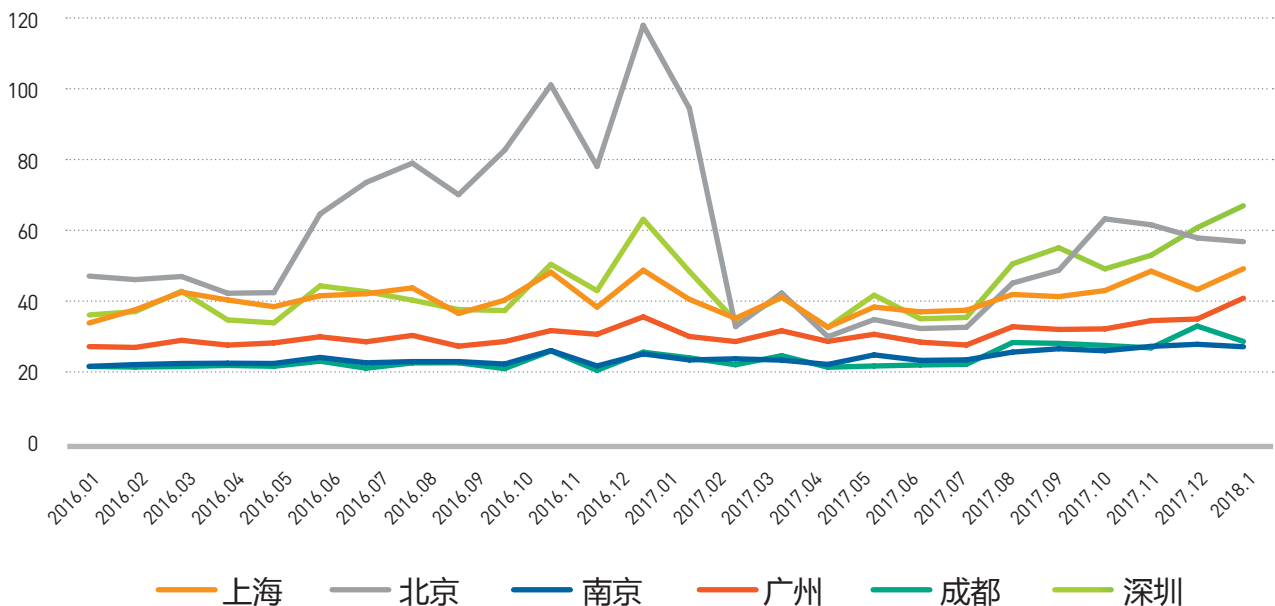
图表 11 - 主要城市新能源汽车产业链供给指数排名——电池供给指数
