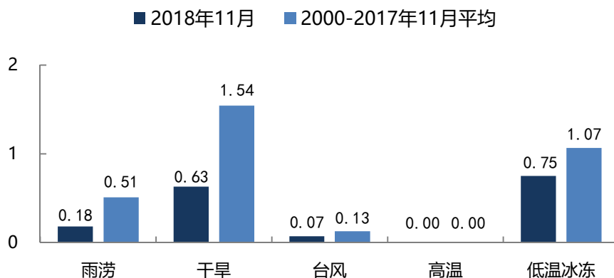
图 2. 2018 年 11 月分项指数
