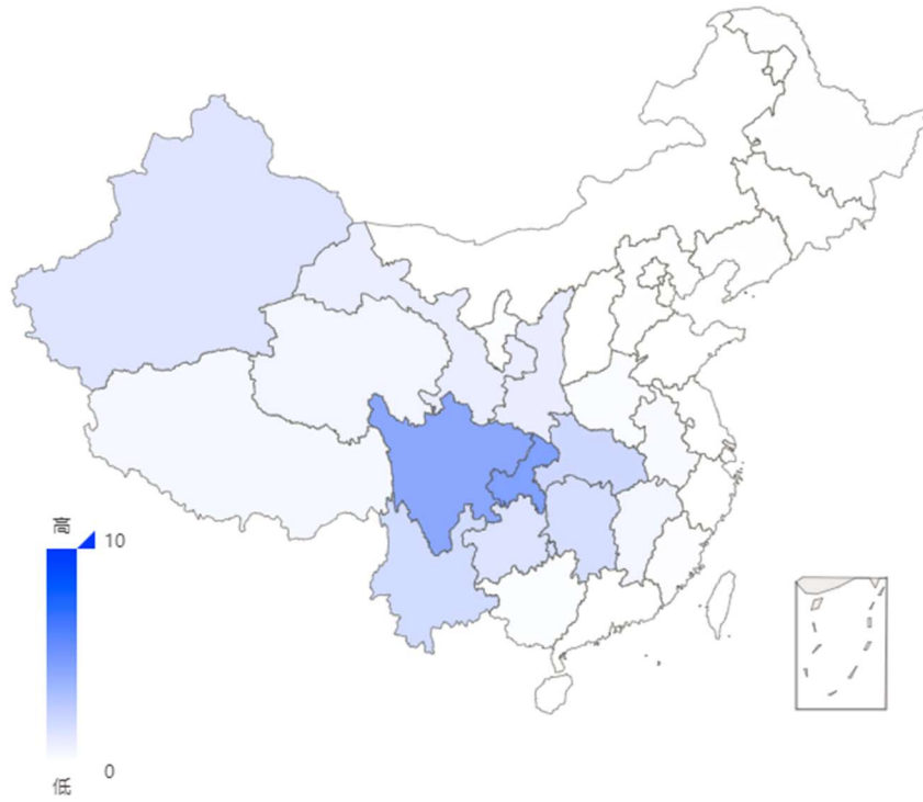
图 4. 2018 年 11 月地区低温冰冻指数监测
